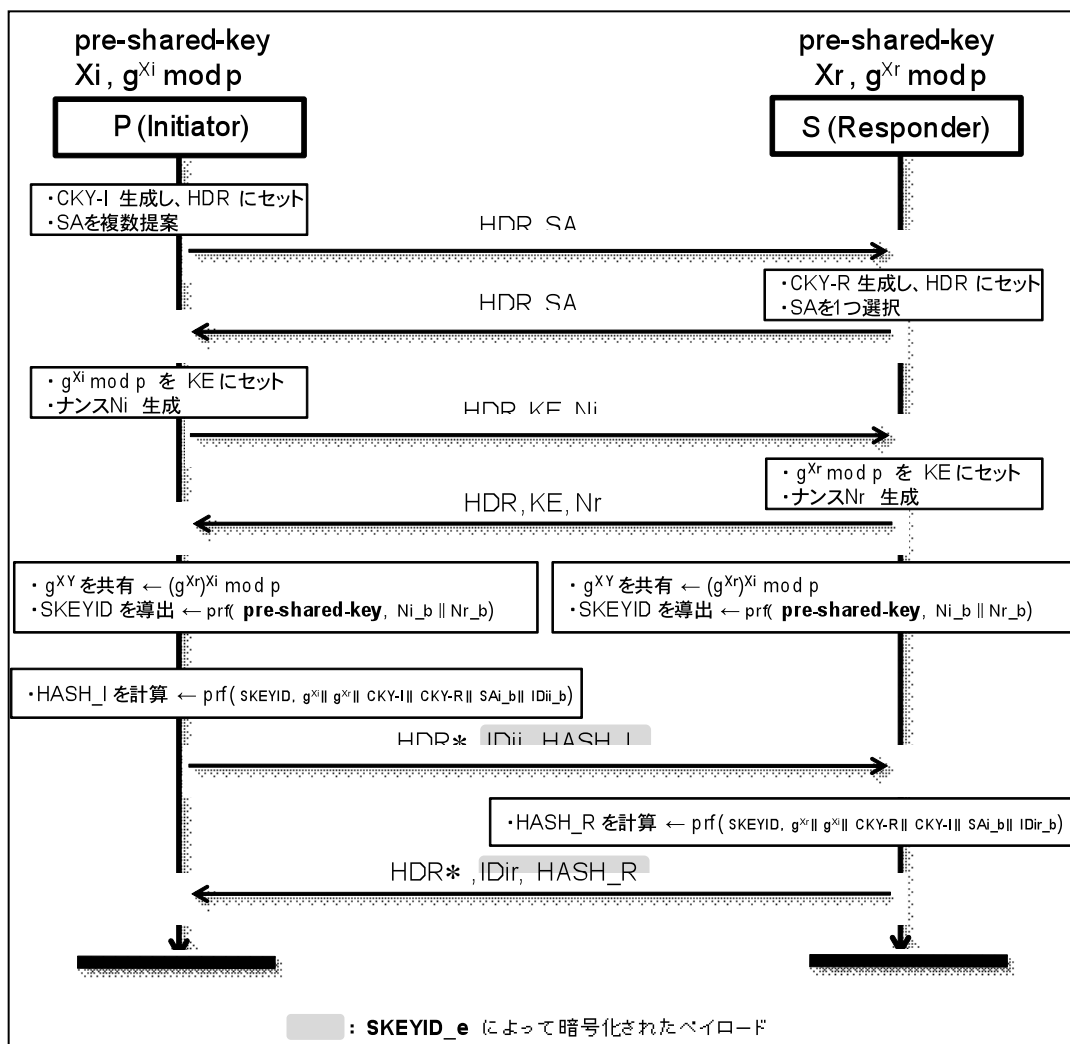
図 1. シーケンス図
